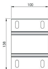
Soporte guía 110x50
