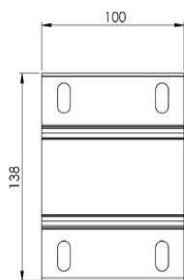
Soporte guía 110*50
