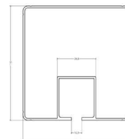
Guía 110x110 (Ver tabla)
