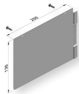
Suplemento tapa tejadillo modular
