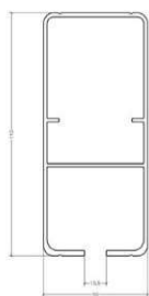
Guía 110*50
