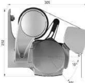
Sist M1 Arko motor pared cerrado- Inclinación- Cotas
