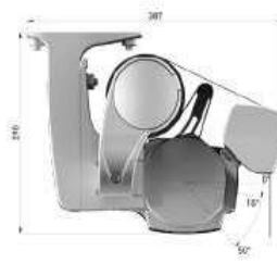
Sist M1 Arko motor techo cerrado- Inclinación- Cotas
