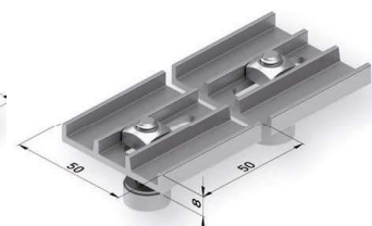
Juego regletas fijación soporte
