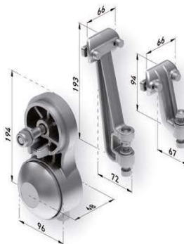
Juego soportes kit cruzado
