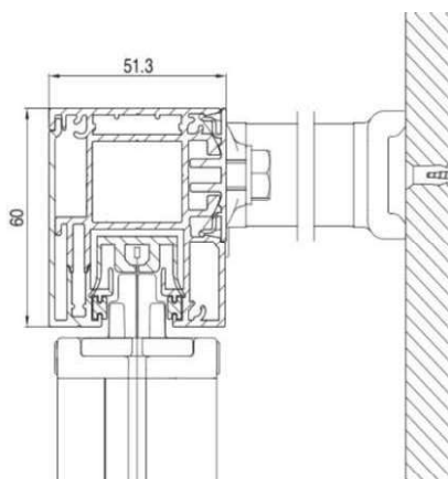
Medidas guía e instalación
