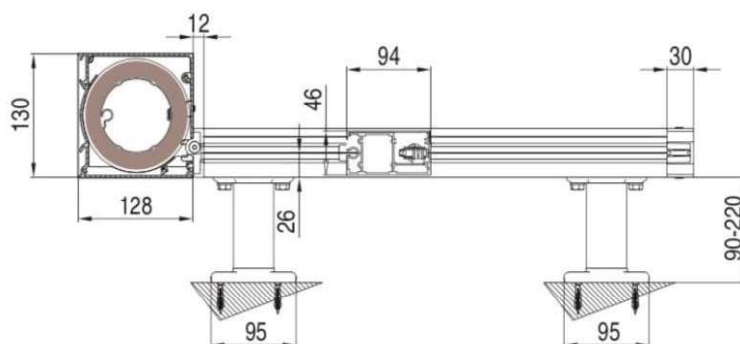
Medidas generales del sistema Tenso Zip Horizontal
